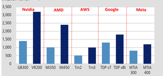
圖 4：AI 晶片熱設計功耗逐代提升，帶動水冷設計升級
