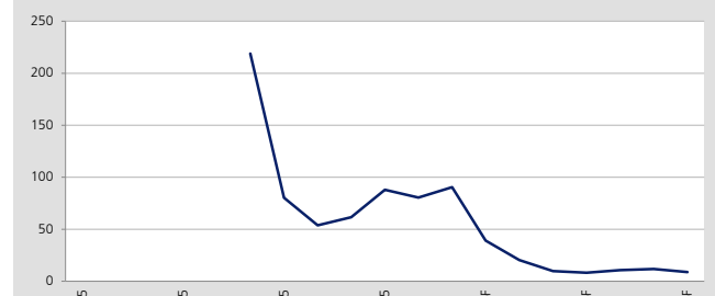
圖 12：本益比
