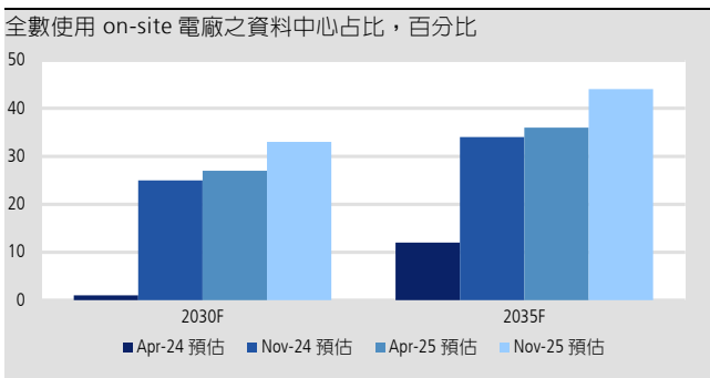
圖 3：資料中心採用 100% on-site 電廠之預期持續提升
